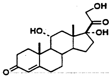
11-Epicortisol
